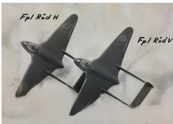
Bild 2. Flygplanens läge i förhållande till varandra i kollisionssögonblicket.
